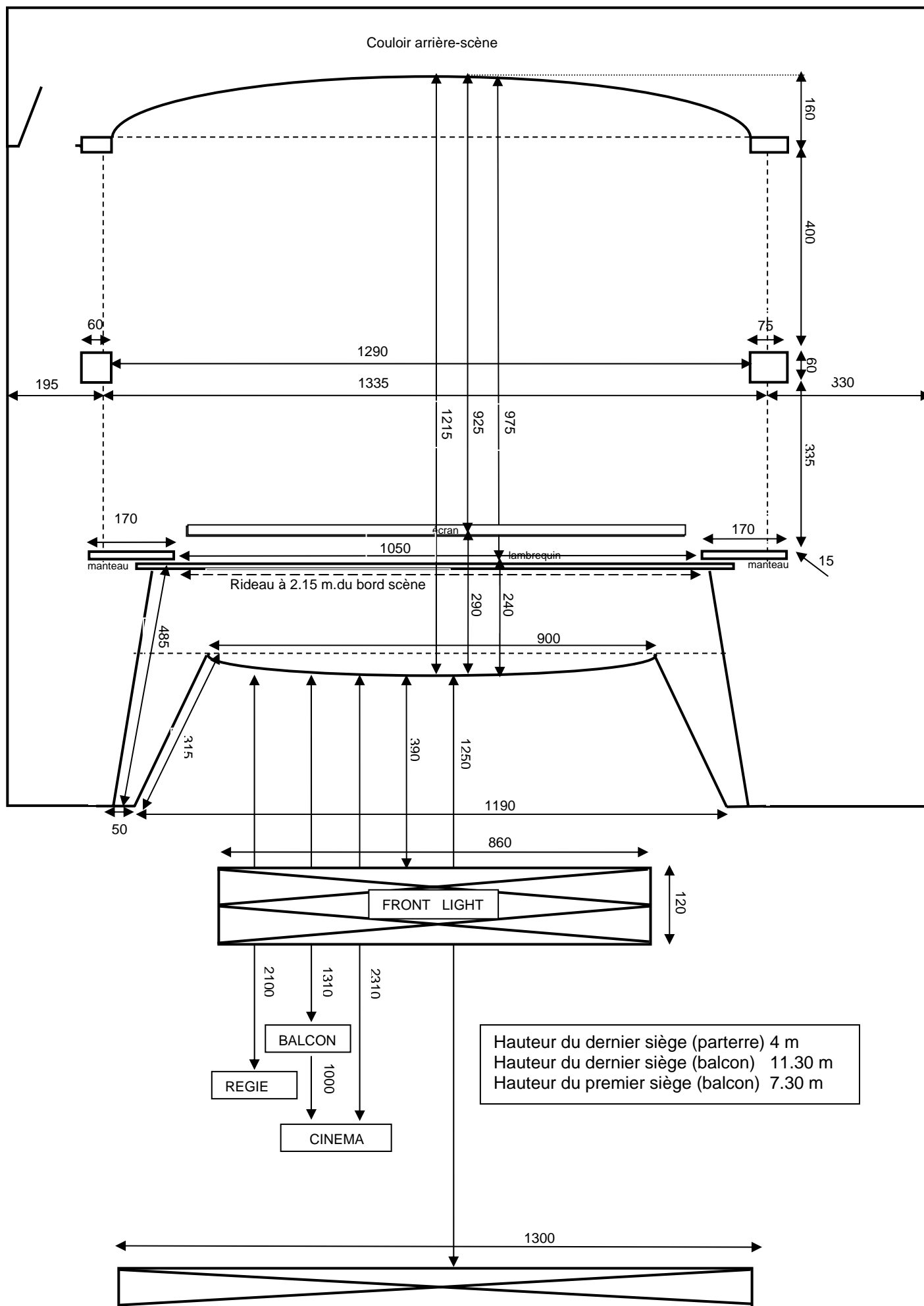
PLAN de SCENE avec ses DIMENSIONS & DISTANCES
